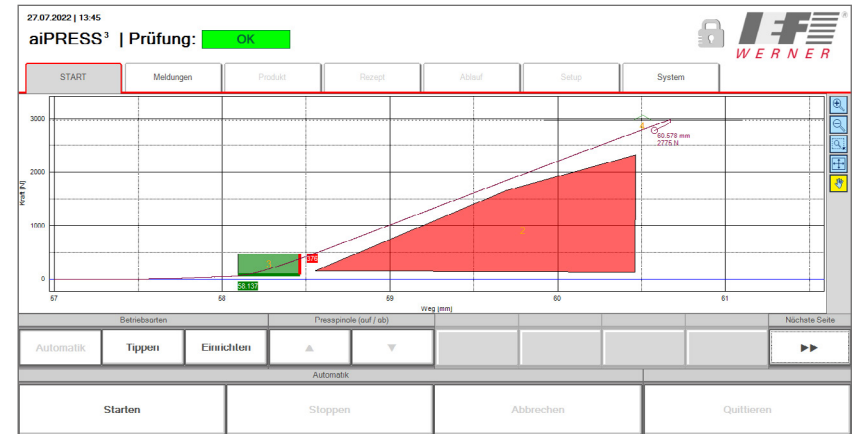
Kraft-Weg Auswertung aiQ-CONTROL (Rezept) Force-path evaluation aiQ-CONTROL (formula)
