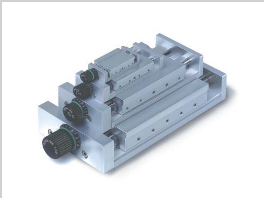
domiLINE 30, 50, 80 und 120 im Größenvergleich domiLINE 30, 50, 80 and 120 sizes
