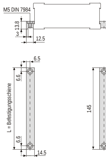
Befestigungssatz B Fastening set B
